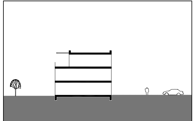
SNEIÐING MKV 1:500
