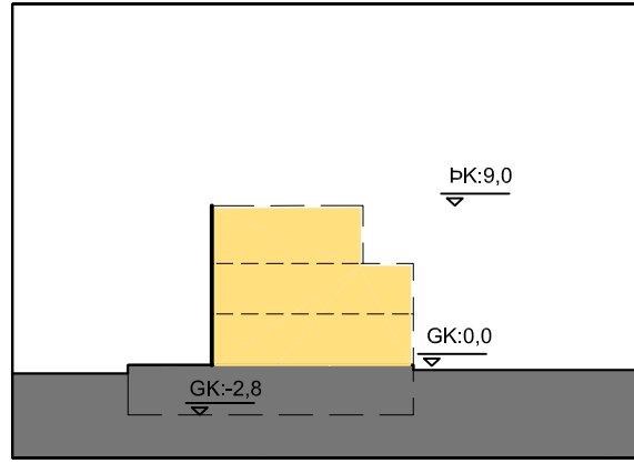
SNEIÐING MKV 1:500
