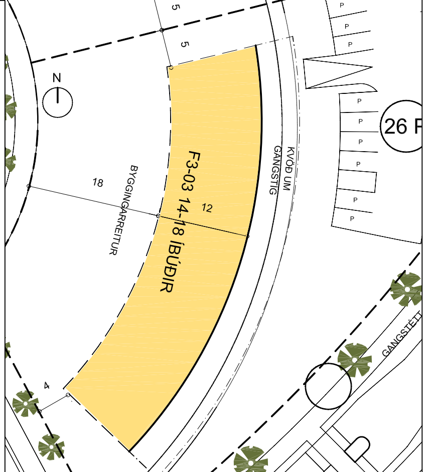
SKILMÁLATEIKNING AF LÖÐ MKV. 1:500
