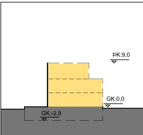
SNEIÐING MKV 1:500
