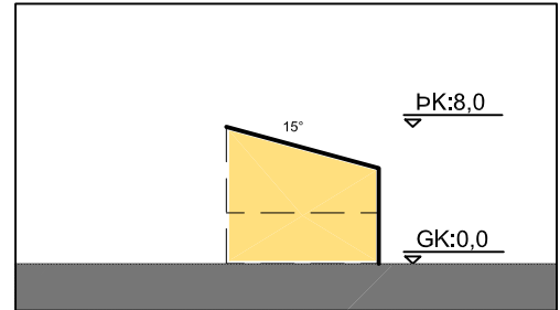
SNEIÐING MKV. 1:500
