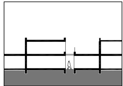
SNEIÐING MKV. 1:500
